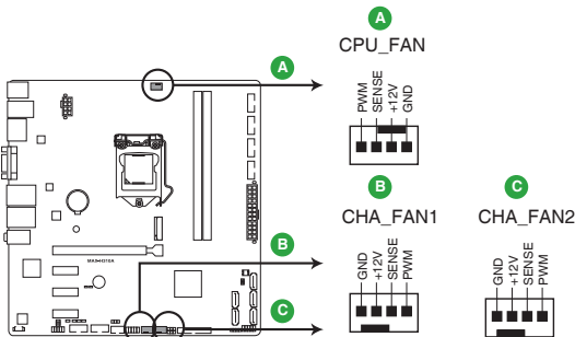
MAX-H310A Fan connectors
