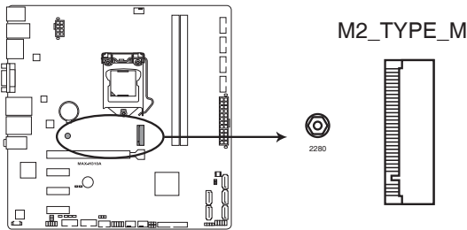
MAX-H310A M.2 (M-key)
